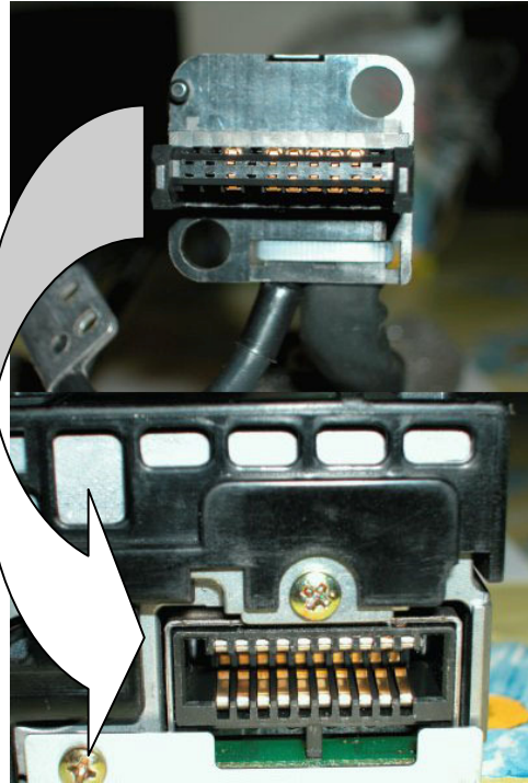
Buchse am Radio in Einbaulage von hinten gesehen und zugehöriger Stecker der Quick-Out-Halterung.
